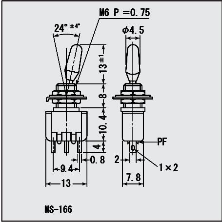
外形図／Dimensions
